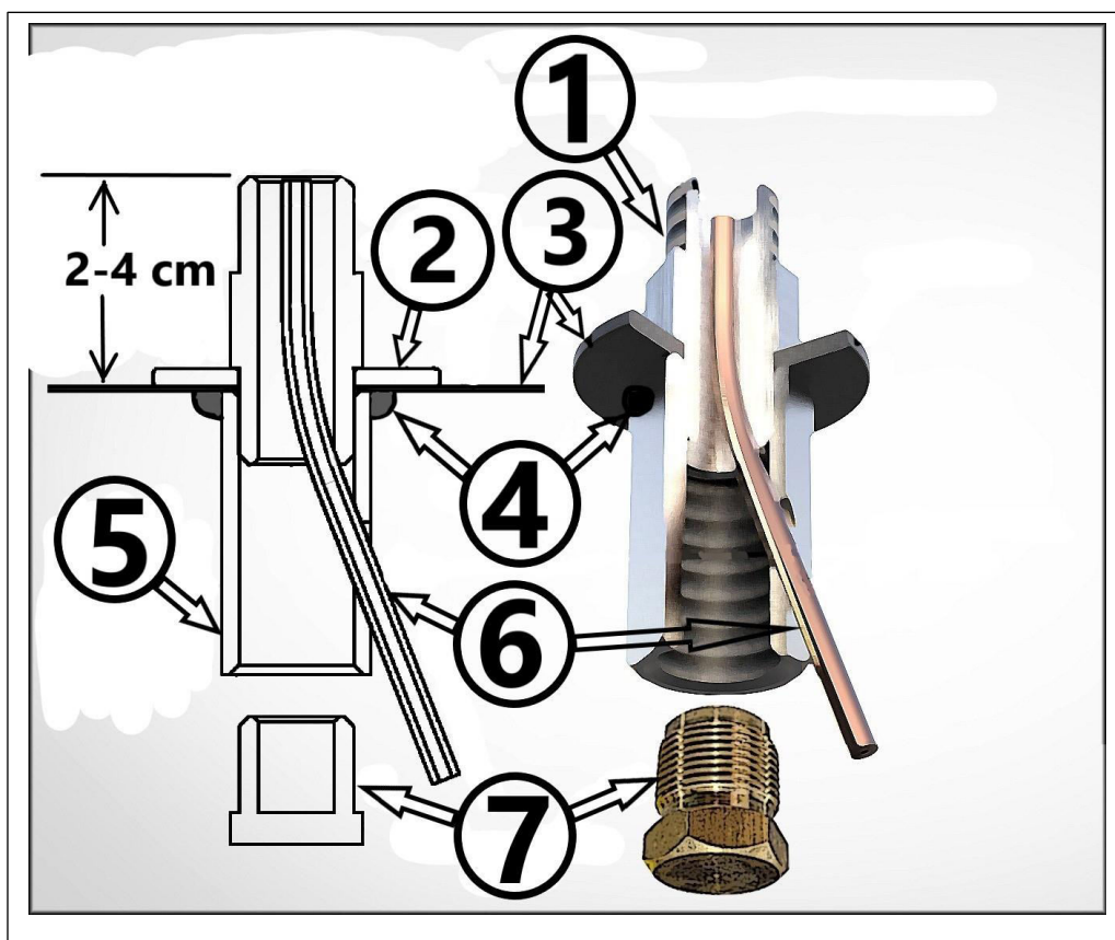
Tobera vista desde adentro del tambor.
